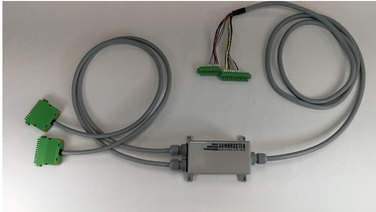
Schrauber-Adapter STAMA-Nr. 3890/ 3893
