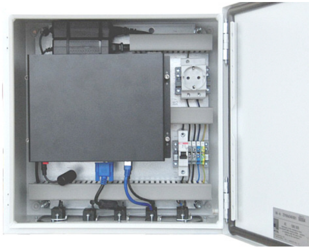
Innenansicht mit eBox-PC 3060 (STAMA Art. Nr. 3274)
